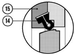
Tätningutförande -85, -86, -8A, -8B
