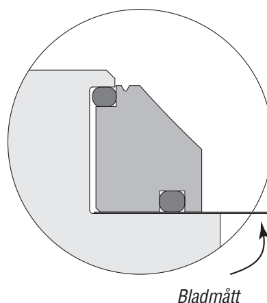
Figur 7. Avluftning med hjälp av bladmått
