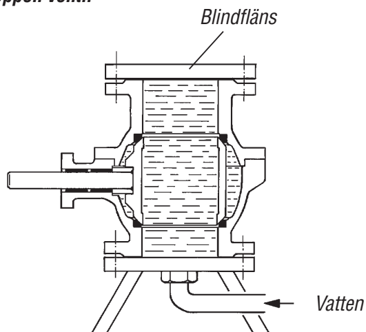
Figur 6. Provning av täthet mellan kulkik och sätesringar
